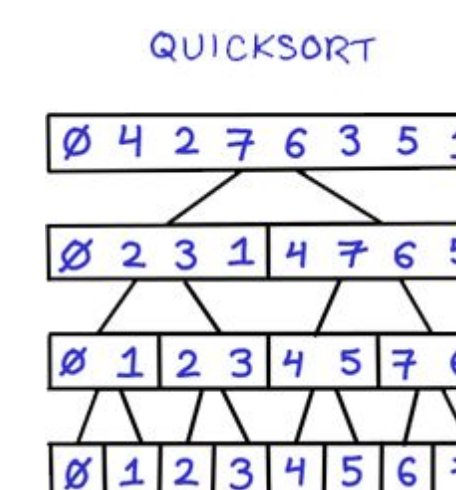
QUICKSORT
