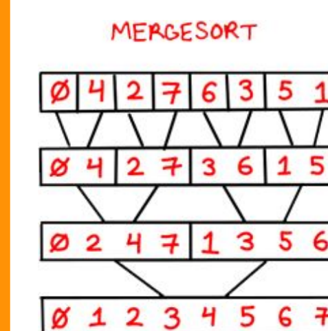
MERGESORT
